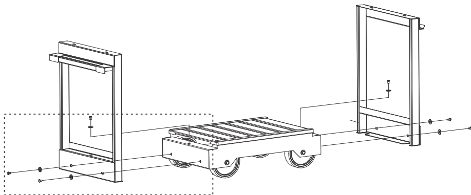
Fig 1 : Coloque los laterales sobre la base y fije los bulones , con sus
