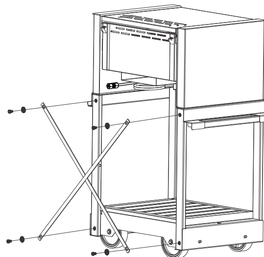
Fig 4 : Coloque de a un tensor a la vez y fije los bulones , con sus arandelas
