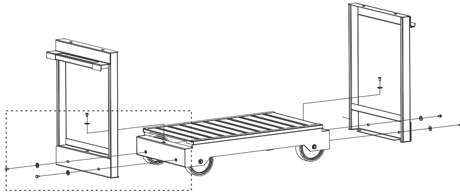
Fig 1 : Coloque los laterales sobre la base y fije los bulones , con sus
