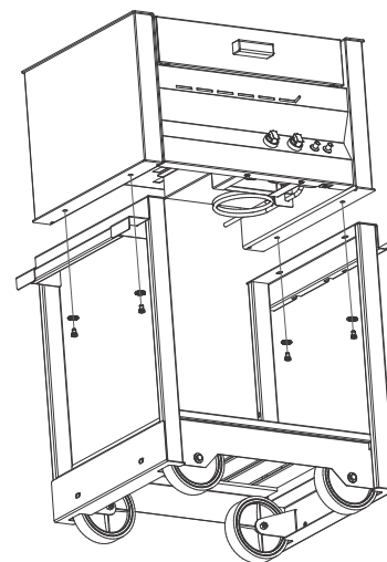
Fig 3 : Coloque el cuerpo de la parrilla sobre la base previamente armada y fije los bulones , con sus arandelas correspondientes, a las tuercas
